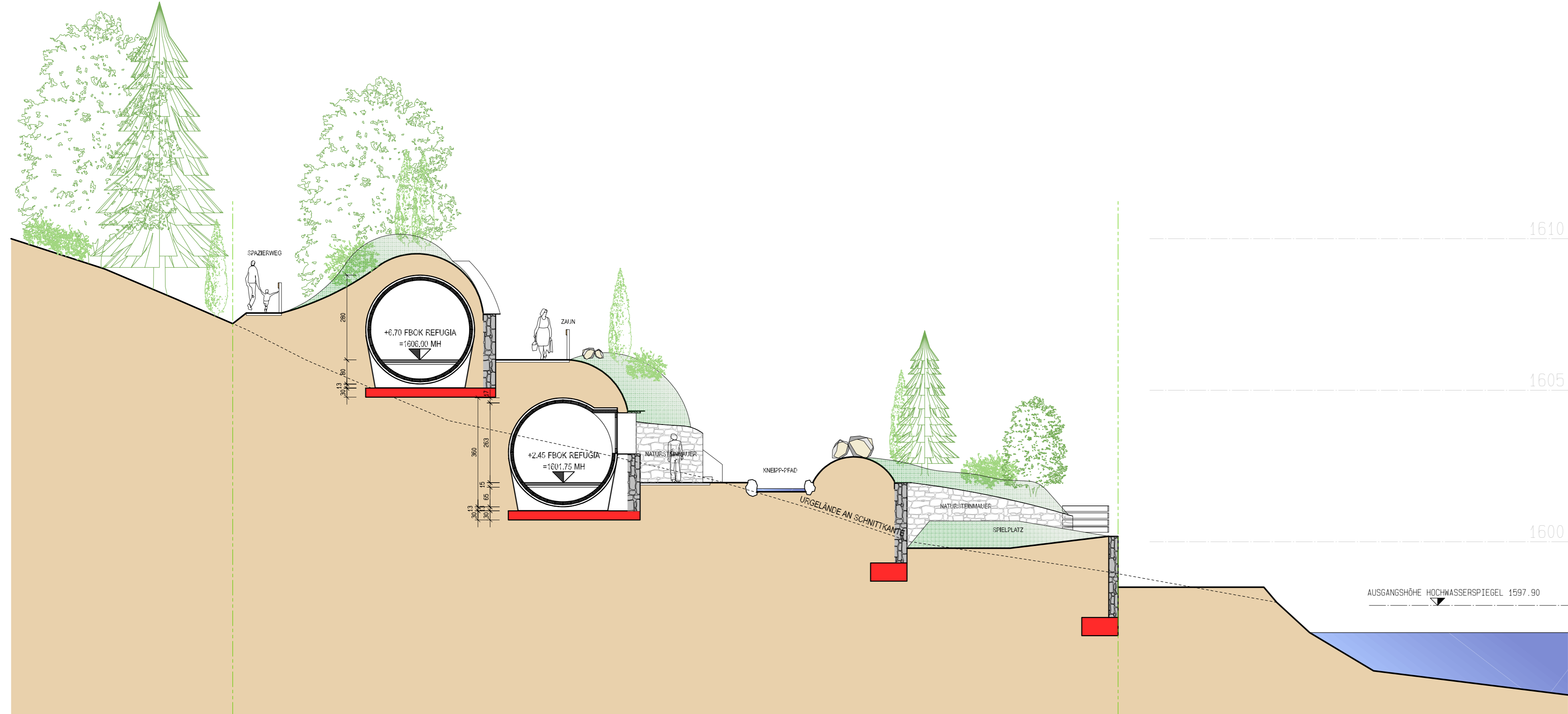
SCHNITT F-F, M 1:100
