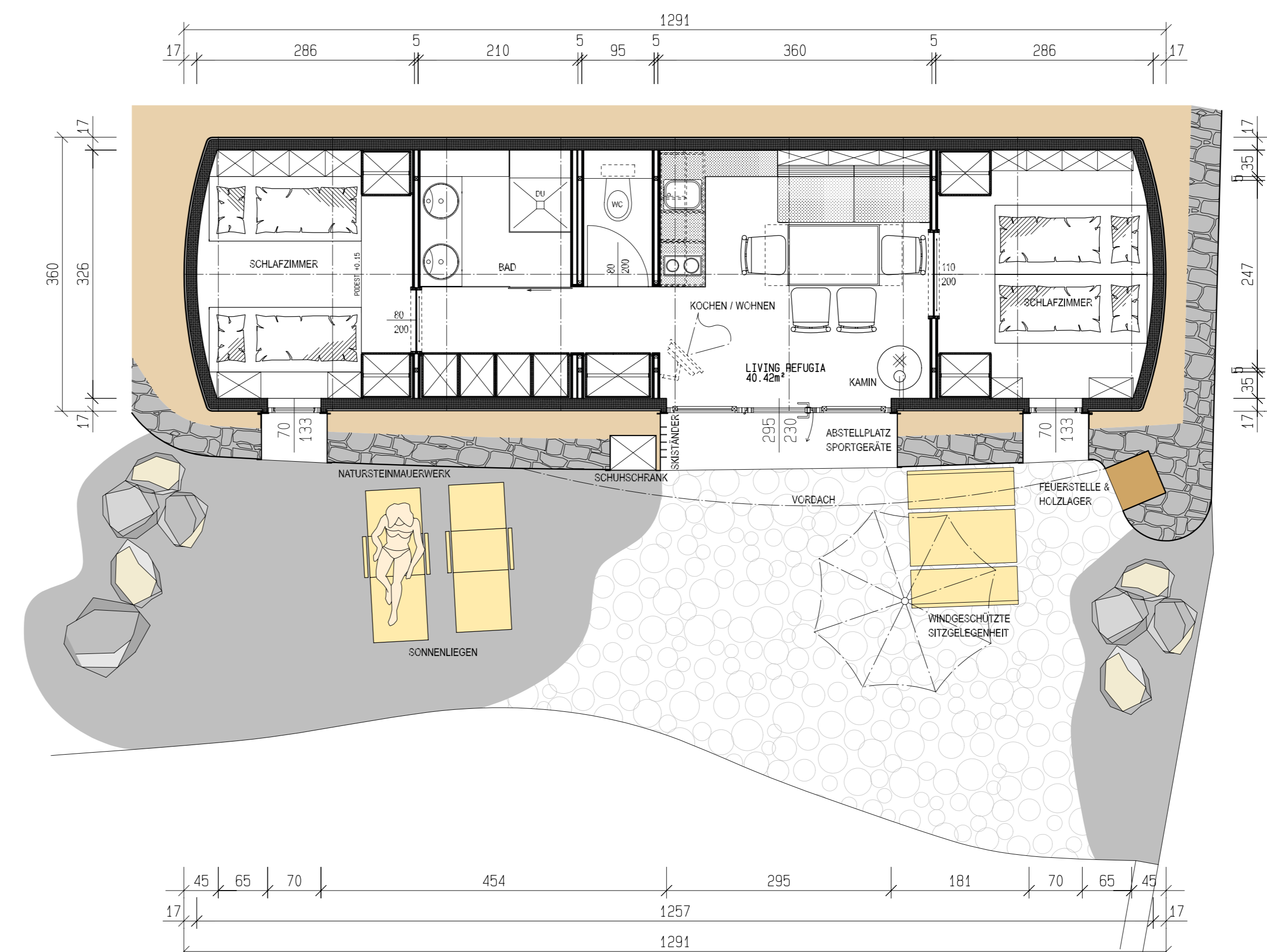
GRUNDRISS LIVING REFUGIA, M 1:50 WOHNEN
