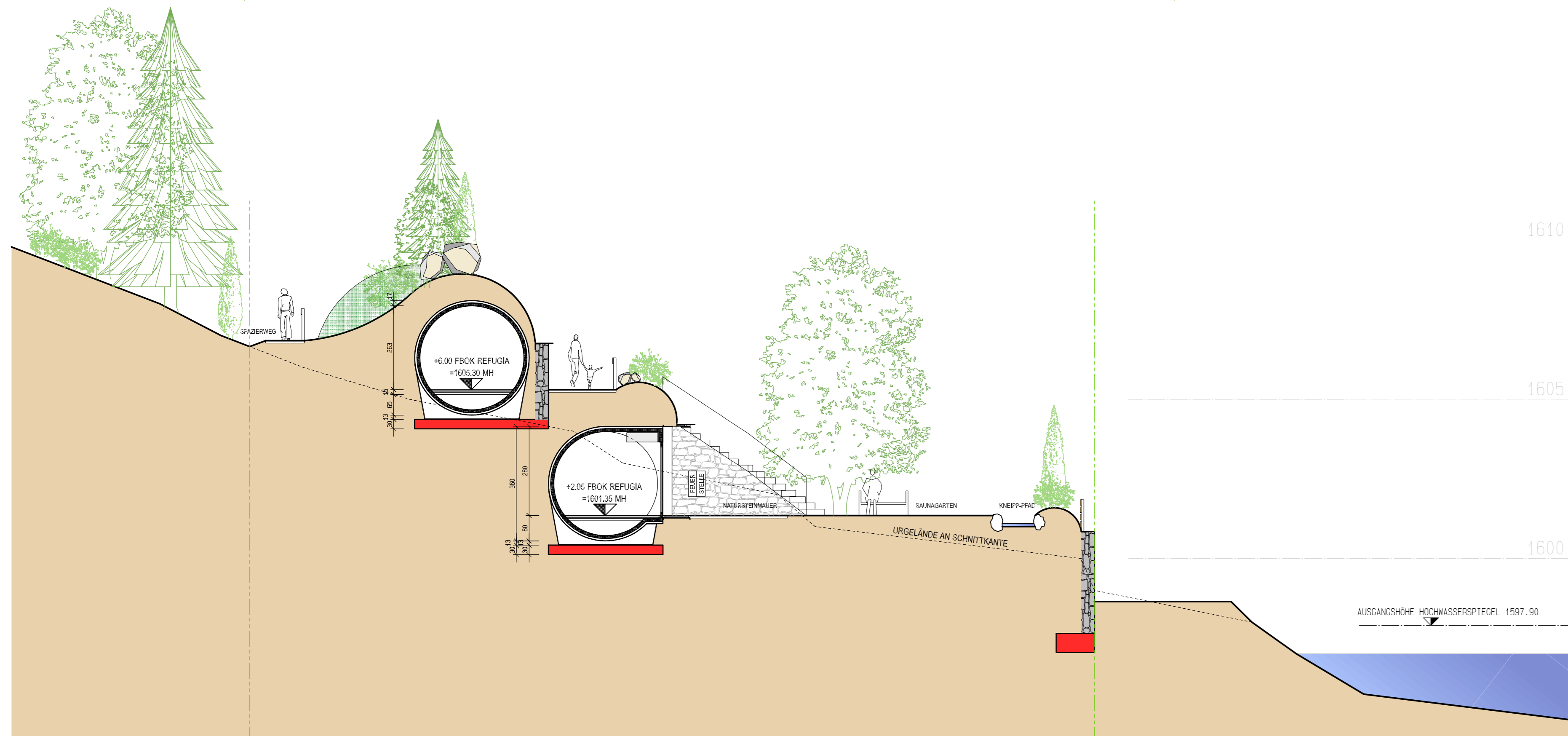
SCHNITT F-F, M 1:100
